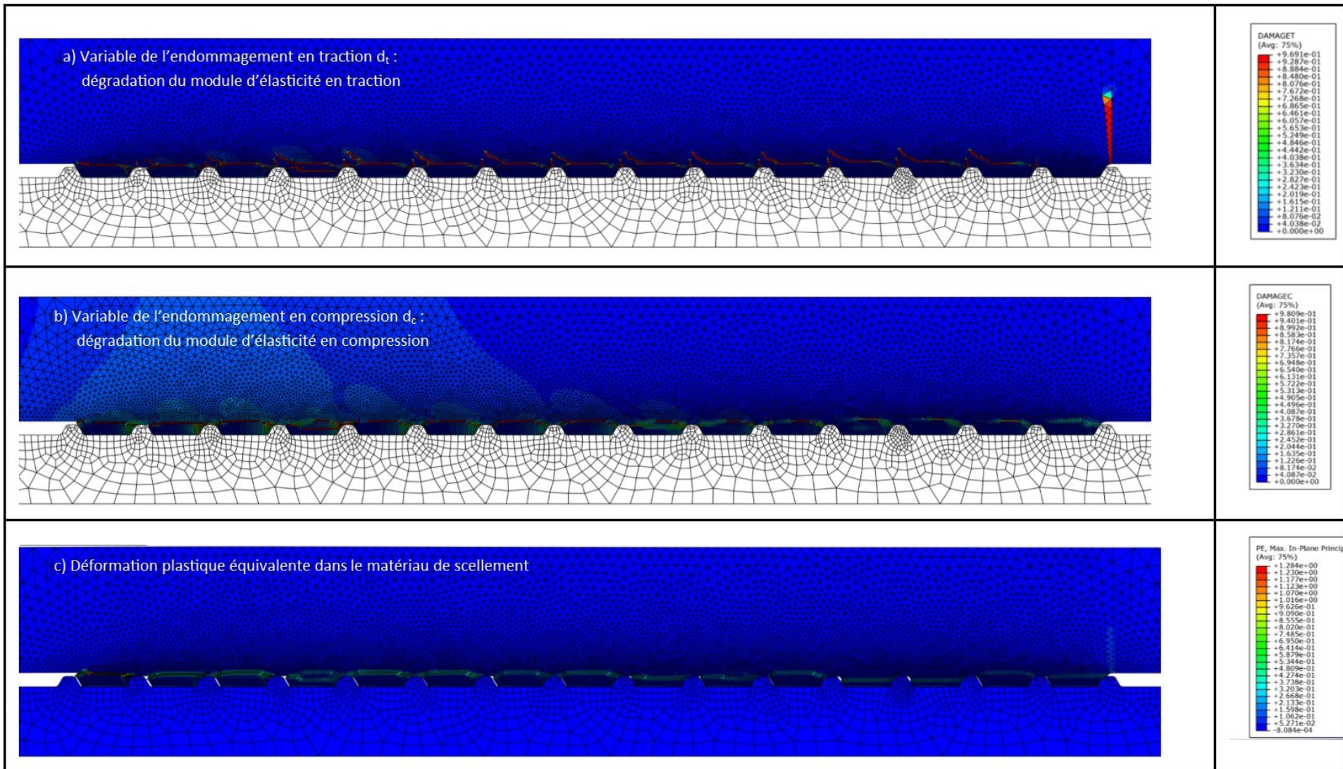
Figure 4 Endommagement et déformation à l'interface barre-scellement
