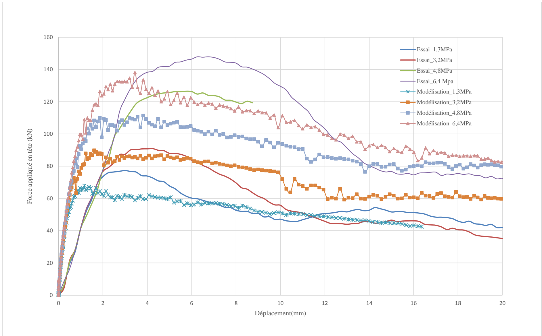
Figure 5 Comparaison entre les résultats de la modélisation numérique et ceux des essais de Moosavi et al (2005) pour différentes contraintes de confinement.
